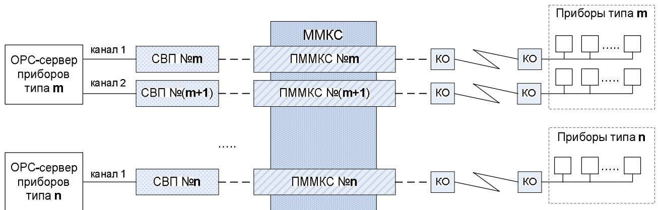
Рисунок 7.1 – Схема взаимодействия ОПС-серверов с устройствами посредством ММКС
