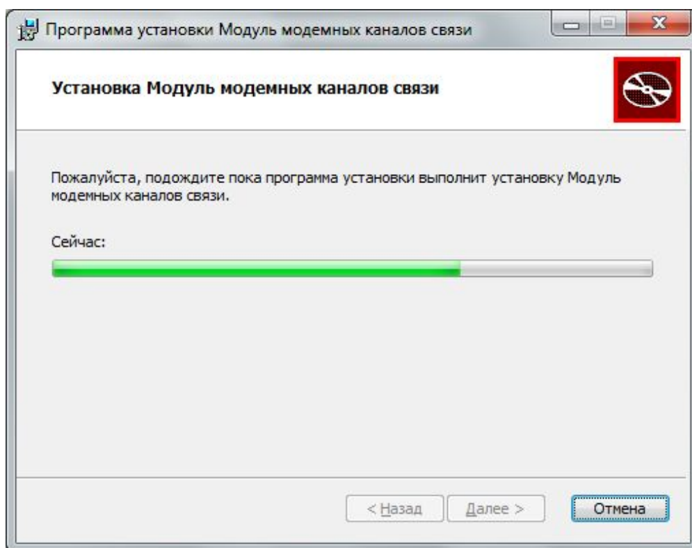
Рисунок 3.5 – Копирование файлов
