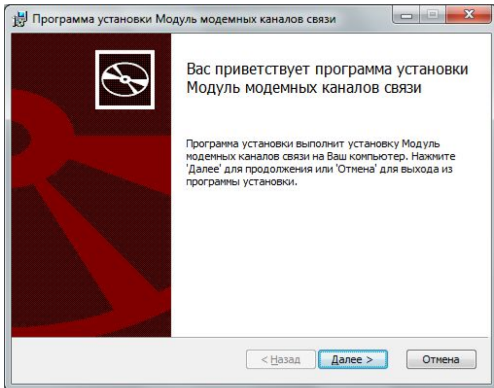
Рисунок 3.1 – Окно инсталлятора
