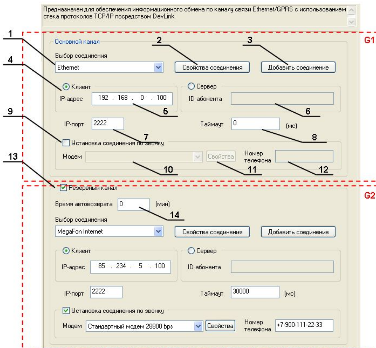
Рисунок П6.1 – Область специфических элементов управления подключаемого модуля «Канал связи DevLink».
