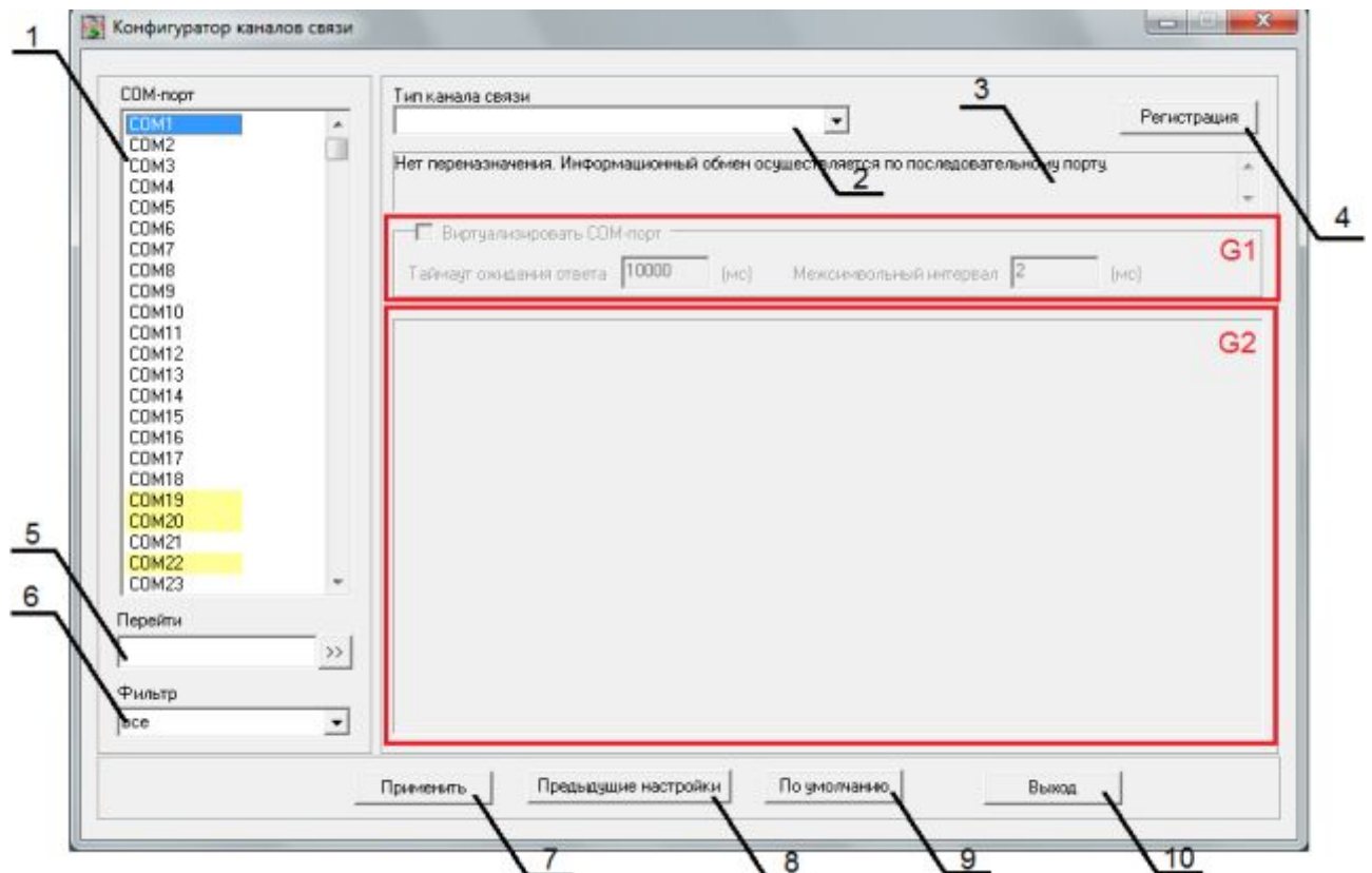
Рисунок 8.1 – Вид окна конфигуратора каналов связи ММКС
