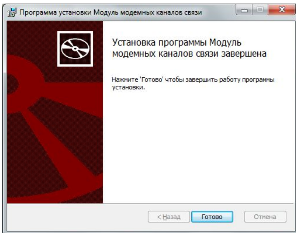
Рисунок 3.6 – Установка завершена
