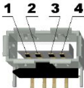
Рисунок 6 – Разъем USBA-1J
