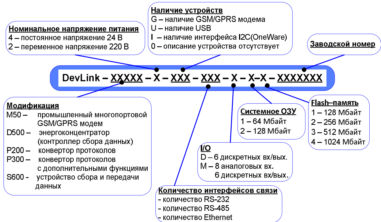
Рисунок 1 – Условное обозначение нестандартных модификаций DevLink®
