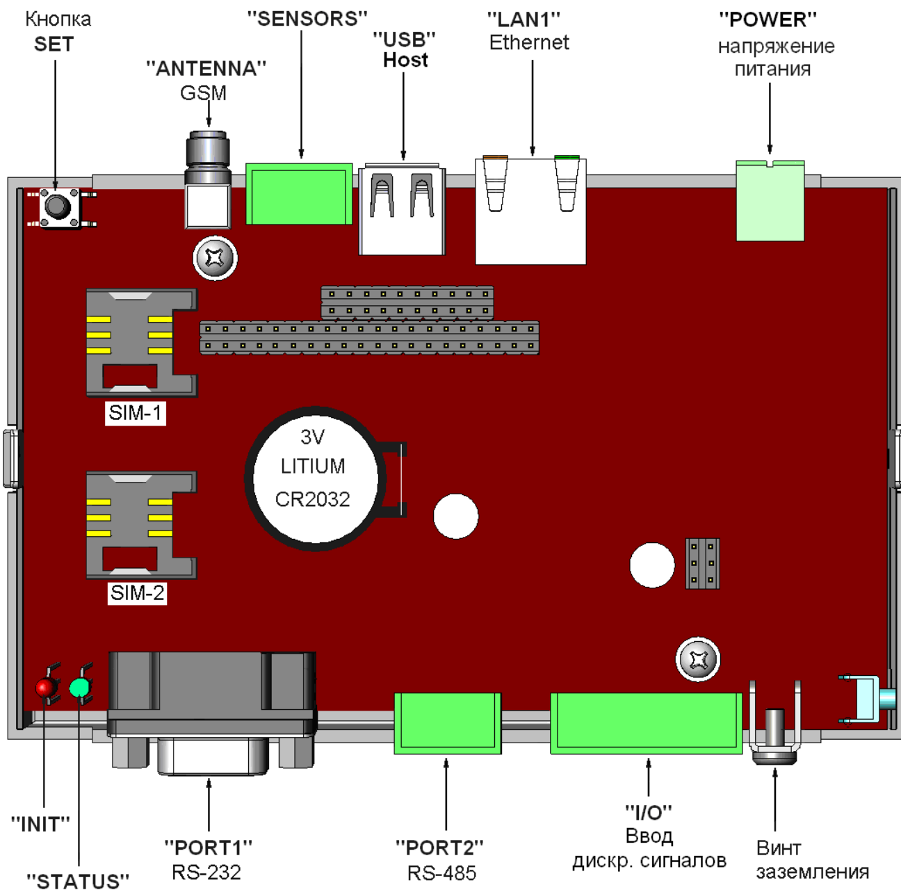
Рисунок 3 – Одноплатный вариант электронного блока DevLink®
