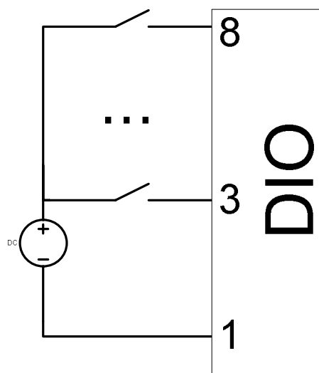
Рисунок 13 – Схема подключения дискретных входов
