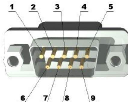
Рисунок 8 – Разъем типа DB-9M (вилка).
